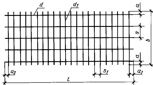
Черт. 1
